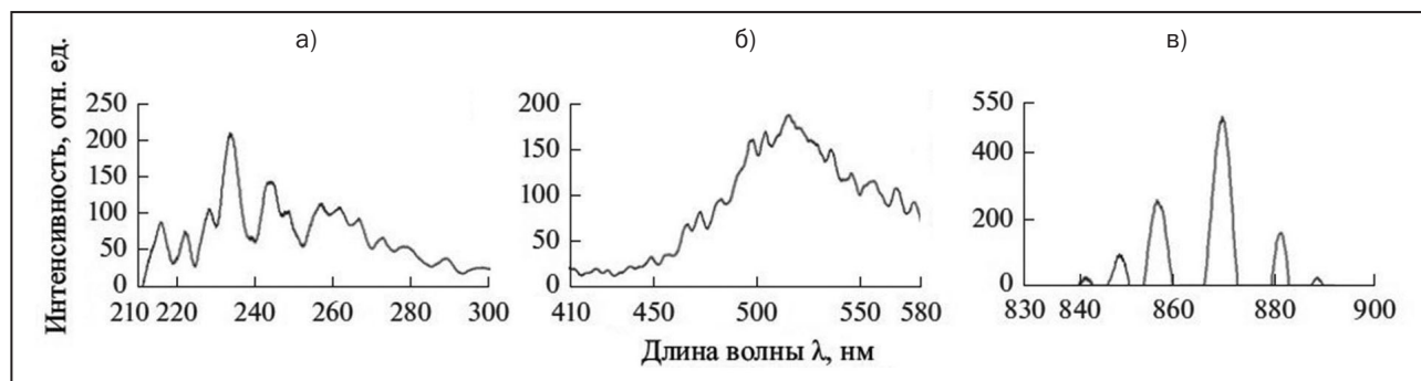
Рис. 2. Типичные спектры люминесценции синтезированных композиционных материалов в зависимости от их состава: а – Cu/Y; б – 2Cu/Y; в – Cu/2Y (на примере \lambda_{\text{возб}} = 200 нм, композиционный материал Cu/Y, термообработка при 870 °С)
