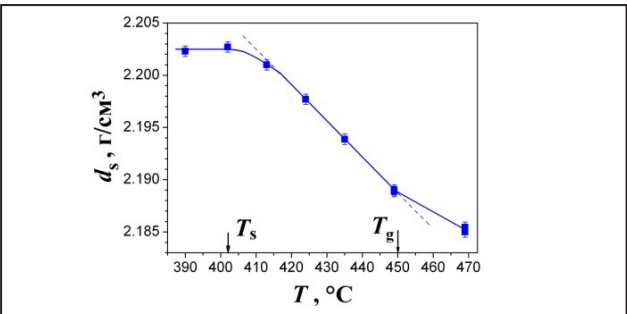
Плотность d s стабилизированного стекла 20Na 2 O·80В 2 О 3 (мол. %) как функция температуры стабилизации. Плотность определялась после охлаждения образца стекла до комнатной температуры. Плотность ниже T g сначала увеличивается с понижением температуры, а затем достигает постоянного значения при T s
