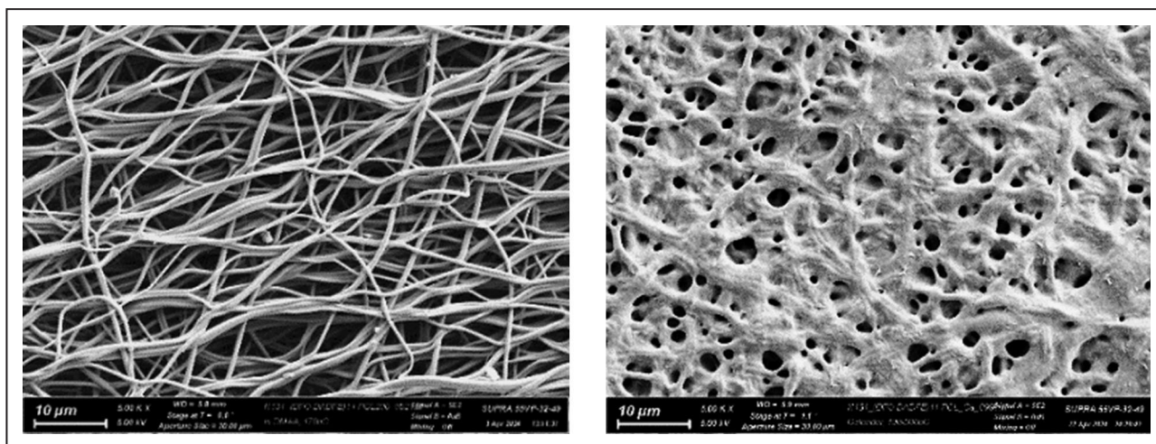
Микрофотографии сканирующей электронной микроскопии образца нетканого СПУИ-материала (слева); того же образца, каландрированного в течение 15 мин при T = 210 °С (справа). Размер пор 0,1–0,05 мкм
